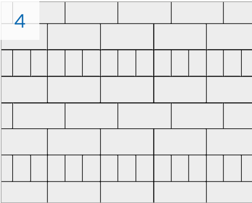
45/30 - 5,56 Stück/m 2 30/15 - 5,56 Stück/m 2
