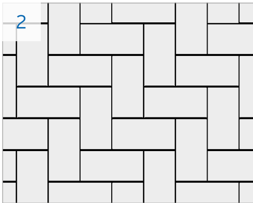
20/10 - 48,00 Stück/m²
