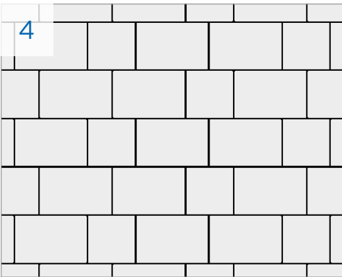
24/16 - 19,53 Stück/m² 16/16 - 9,77 Stück/m²
