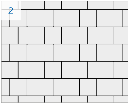
21/14 - 25,51 Stück/m² 14/14 - 12,76 Stück/m²
