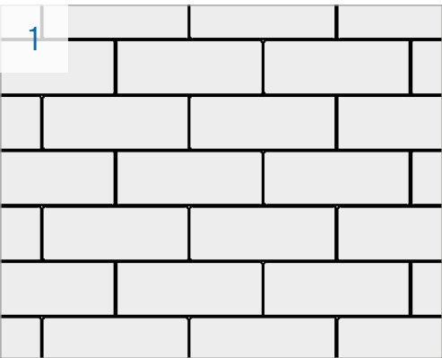
20/10 - 48,00 Stück/m²
