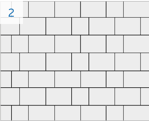
24/16 - 21,31 Stück/m² 16/16 - 7,10 Stück/m²
