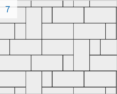
30/20 - 2,38 Stück/m² 60/30 - 4,76 Stück/m²
