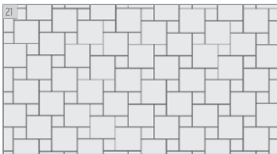
21 Versetzter Verband
