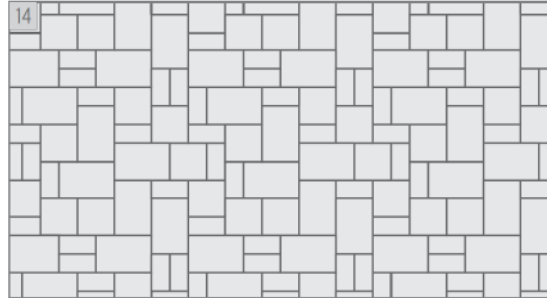
14 Wechsverband B 45 x 30 cm 30 x 20 cm 30 x 30 cm oder 20 x 20 cm 30 x 15 cm 10 x 20 cm
