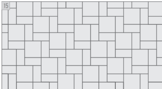
15 Wechsverband C 30 x 30 cm oder 20 x 20 cm 30 x 15 cm oder 20 x 10 cm
