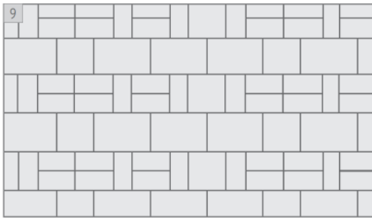
9 Gleichmäßiger Verband A
