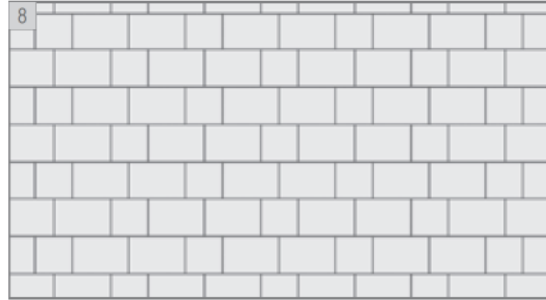
8 Gleichmäßiger Reihenverband B
