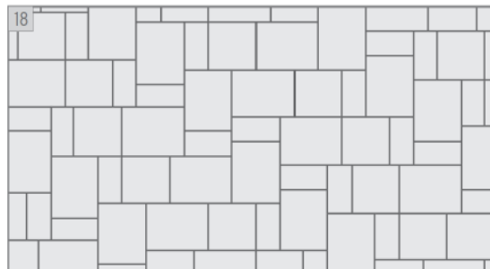
18 Wilder Verband A 45 x 30 cm 30 x 20 cm 30 x 30 cm oder 20 x 20 cm 30 x 15 cm 10 x 20 cm
